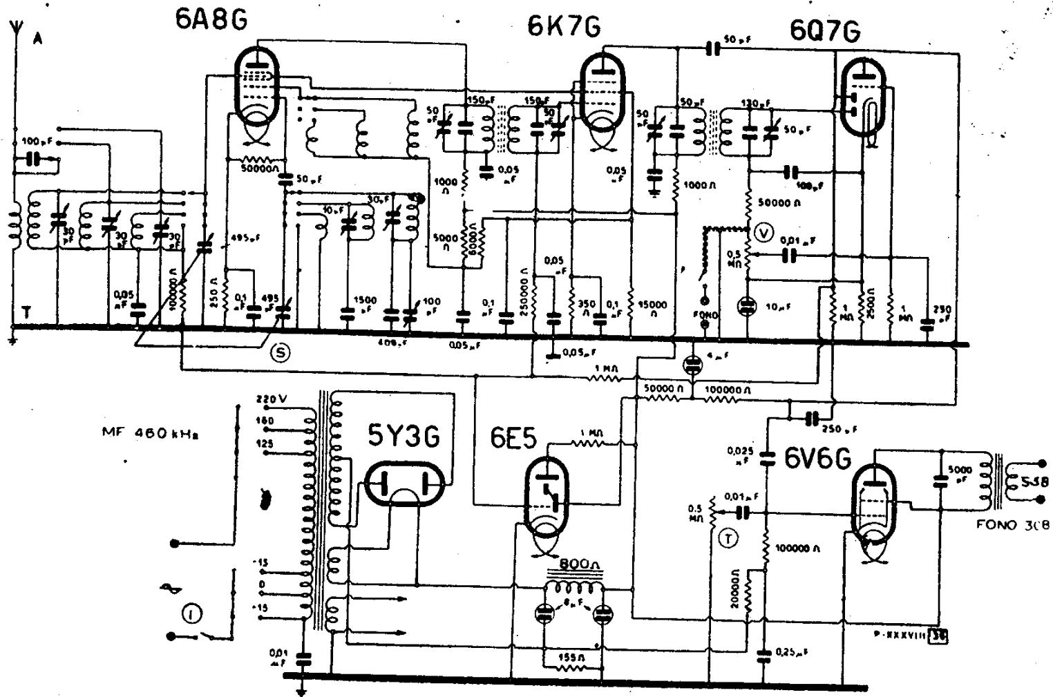
WATT RADIO - MOD « AUTOSINTON »
